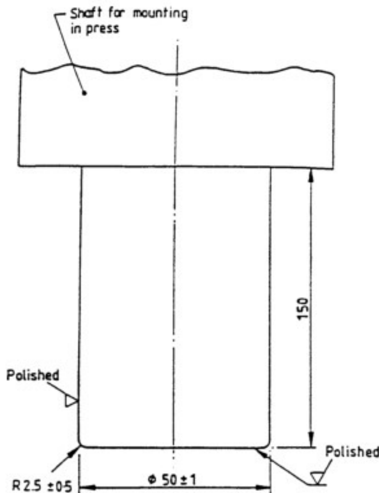
FIG. 1 Plunger
